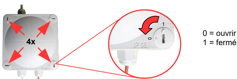
Illustration 4: Retirez le couvercle du boîtier de commande du capteur .
