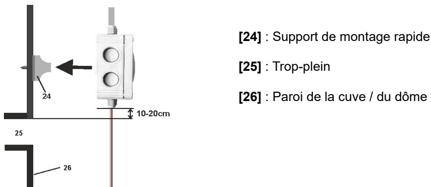
Illustration 8: Placez le transducteur sur le support de montage rapide .
