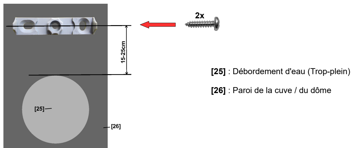
Illustration 6: Vissez le support de montage rapide.
